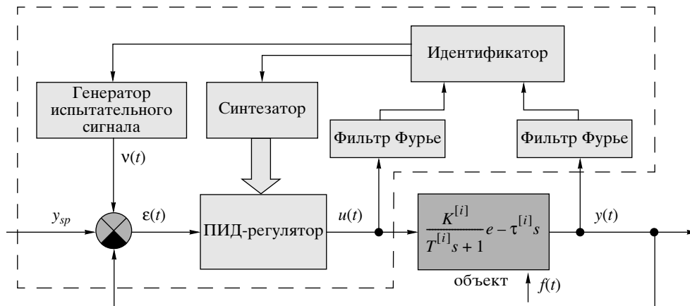
Рис. 1. Структурная схема системы с частотным адаптивным ПИД-регулятором.
